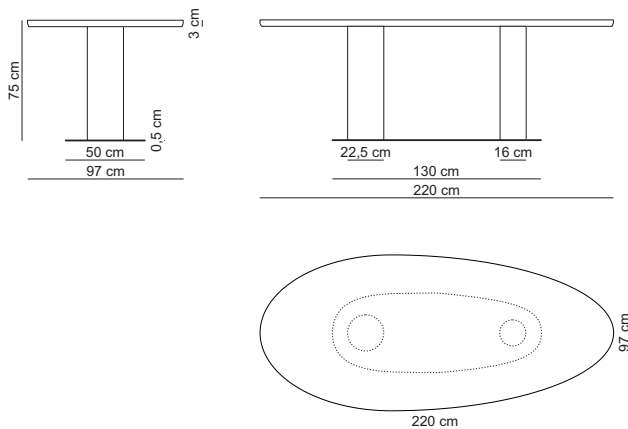
220x75x97 high / 220X97H
