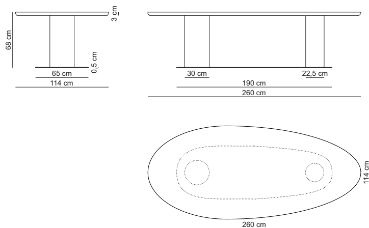
260x68x114 low / 260X114L
